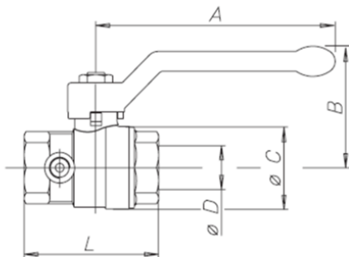
Габаритные и присоединительные размеры
