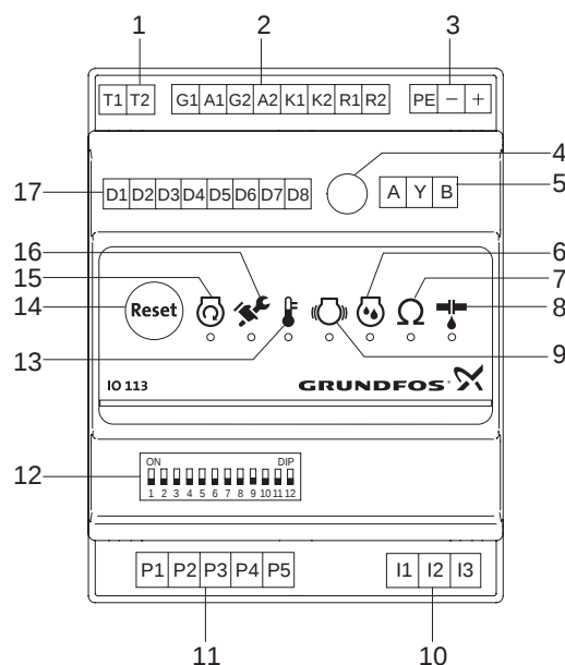
Рис. 154 Модуль IO 113
