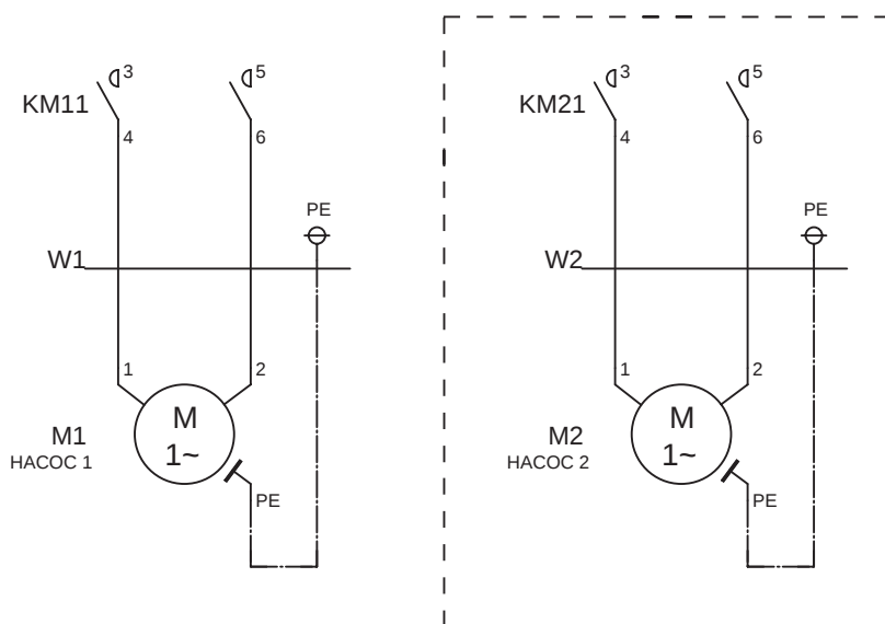
Рис. 46 Подключение однофазных насосов с конденсаторами
