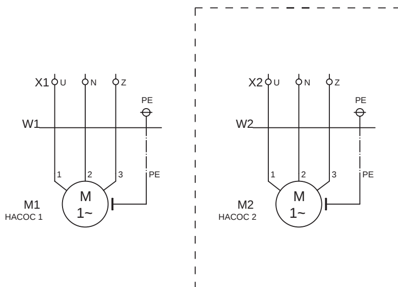
Рис. 47 Подключение однофазных насосов без конденсаторов (конденсаторы в составе шкафа)
