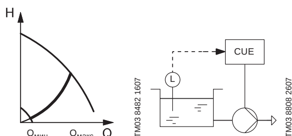
Рис. 95 Постоянный уровень
