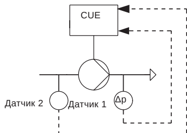
Рис. 90 Перепад давления от двух датчиков
