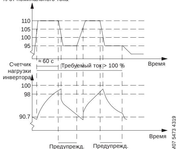
Рис. 114 Выходной ток в условиях перегрузки
