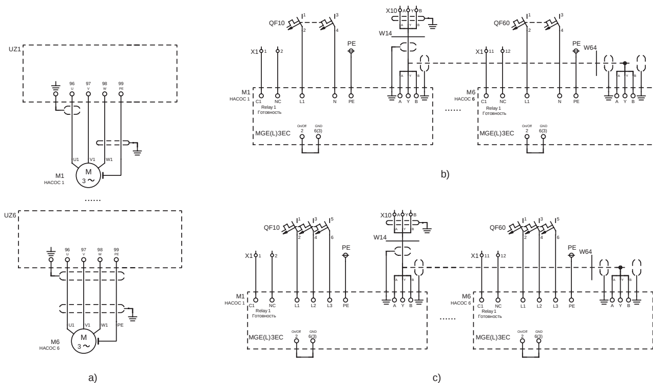
Рис. 38 Подключение насосов по схеме: а) через преобразователи частоты в шкафу (ESS); б) через преобразователи частоты на насосах 1х220В; в) через преобразователи частоты на насосах 3х380 В
