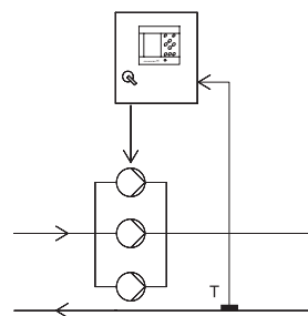
Рис. 18 Температура в обратном трубопроводе
