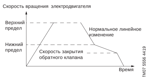
Рис. 123 Контроль скорости закрывания обратного клапана
