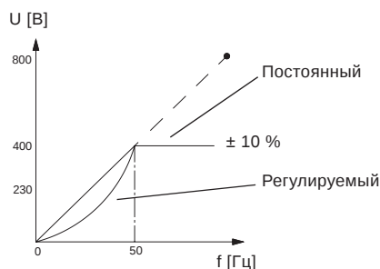
Рис. 112 Регулирование по характеристике U/f (идеальное)
