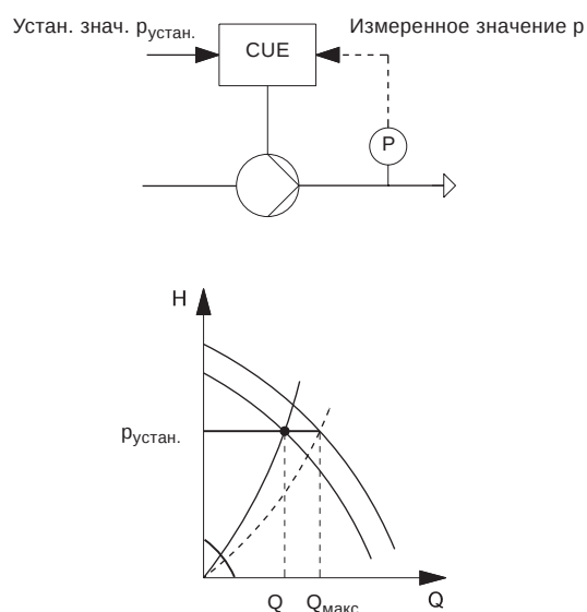
Рис. 106 Регулирование по постоянному давлению
