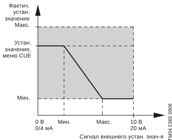
Рис. 103 Сокращённый обратный сигнал внешнего установленного значения
