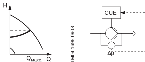
Рис. 92 Перепад давления, параболическая кривая
