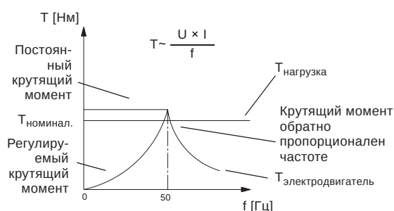
Рис. 113 Регулирование по характеристике T/п (идеальное)
