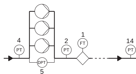
Рис. 22 Повышение давления
