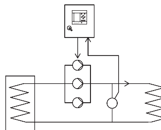
Рис. 7 Циркуляционная система
