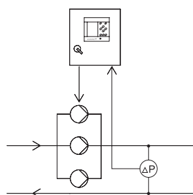
Рис. 15 Перепад давления
