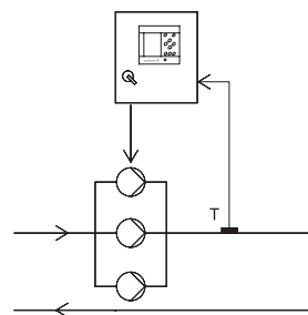
Рис. 17 Температура в напорном трубопроводе
