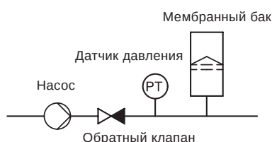
Рис. 87 Расположение обратного клапана и датчика давления в системе, имеющей подпор на входе
