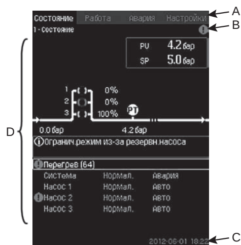
Рис. 12 Структура дисплея
