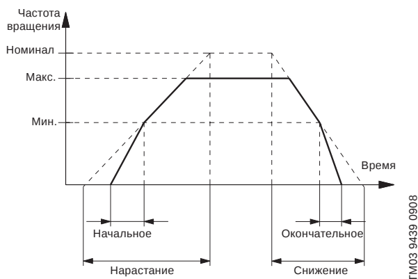
Рис. 119 Нарастание и снижение CUE
