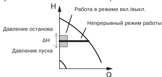
Рис. 85 Постоянное давление с функцией останова. Разница между значениями давления пуска и останова ( \Delta H )
