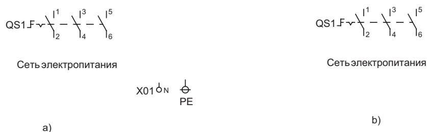
Рис. 35 Один ввод питания: а) 3х380V, N, PE для шкафов с общим потребляемым током до 55 А; б) 3х380V, PE для шкафов с общим потребляемым током более 55 А
