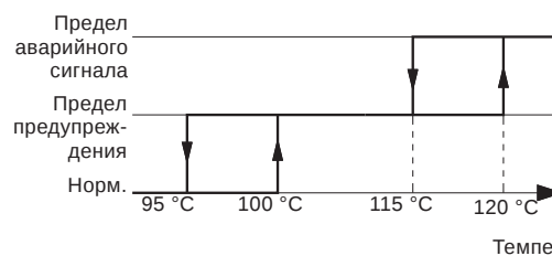
Рис. 124 Контроль температуры подшипников с использованием предельных значений для предупреждений и аварийных сигналов
