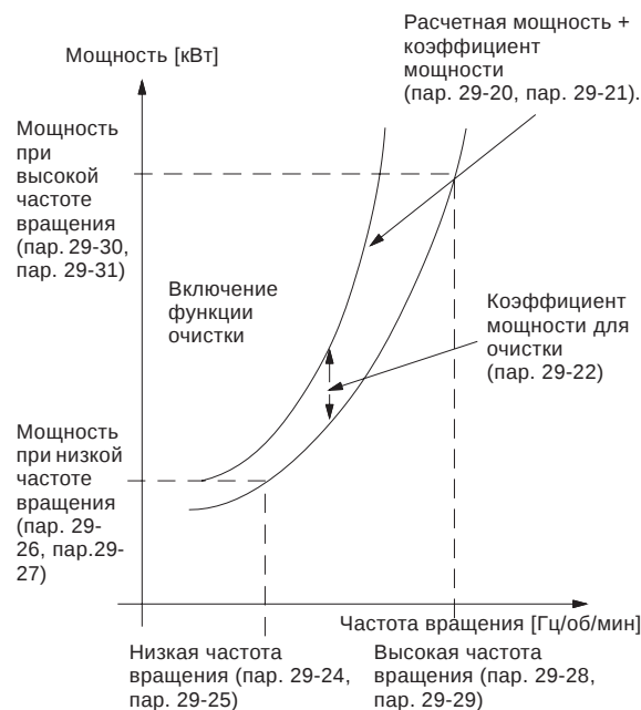
Рис. 122 Регулировка мощности для очистки
