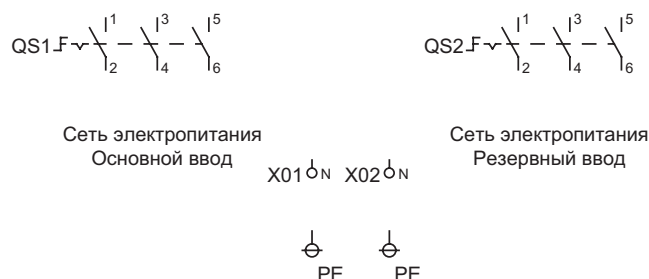
Рис. 36 Двойной ввод питания 3х380V, N, PE с ABP
