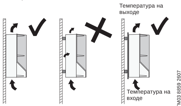
Рис. 126 Вешайте CUE непосредственно на стену или устанавливайте на крепежную пластину с проставками
