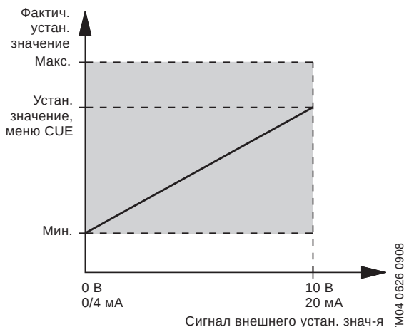
Рис. 100 Внешнее установленное значение
