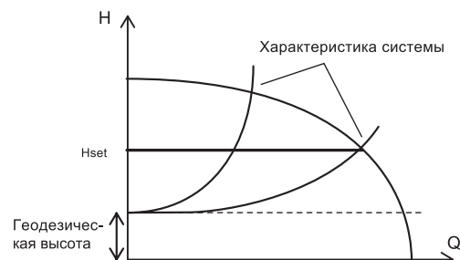
Рис. 6 Характеристика установки повышения давления
