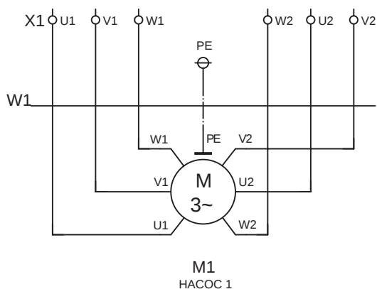
Рис. 50 Подключение трехфазных насосов по схеме «звезда-треугольник» (SD)
