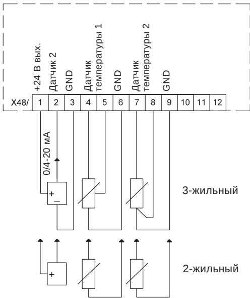
Рис. 143 Схема электрических соединений, MCB 114
