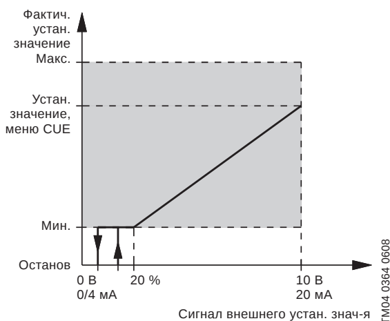
Рис. 104 Внешнее установленное значение с функцией останова
