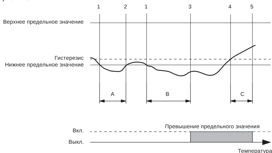
Рис. 125 Пример превышения нижнего предела
