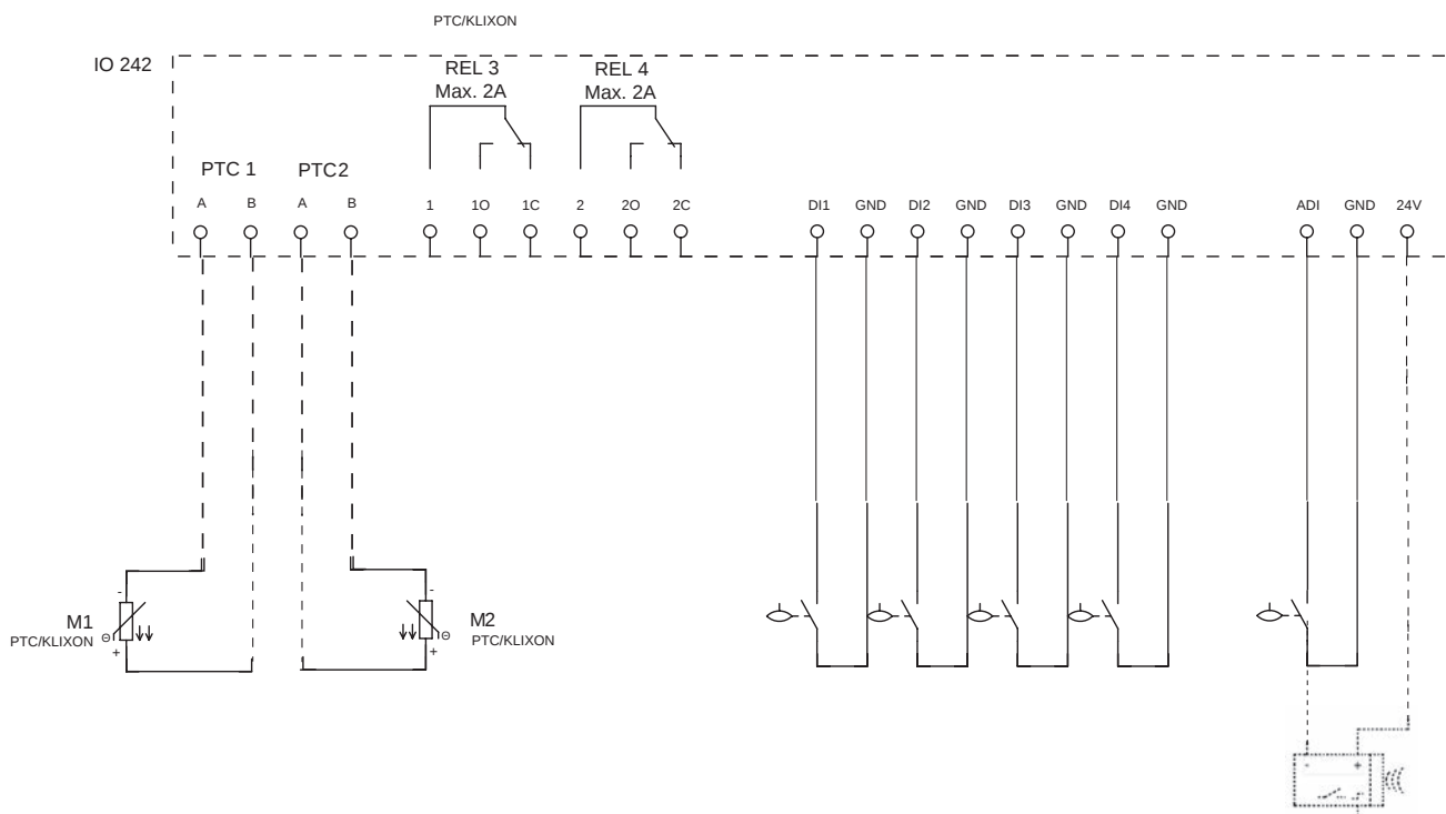
Рис. 54 Подключение сигнальных цепей. Шкаф управления двумя насосами
