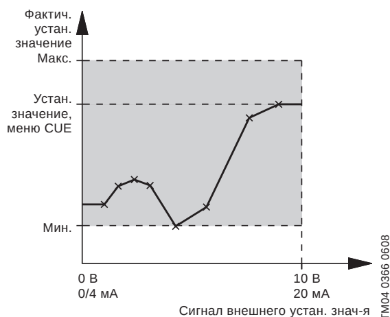
Рис. 105 Внешнее установленное значение по справочной таблице
