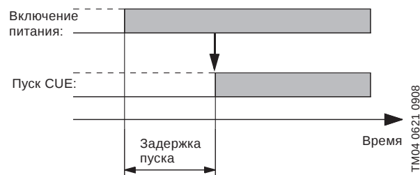
Рис. 115 Задержка пуска после включения питания
