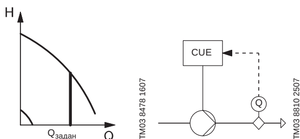
Рис. 94 Постоянный расход
