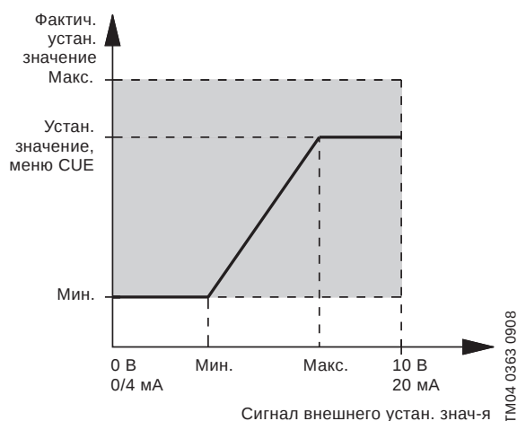
Рис. 101 Сокращённый сигнал внешнего установленного значения
