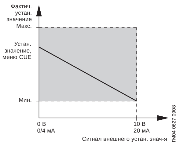
Рис. 102 Обратный сигнал внешнего установленного значения
