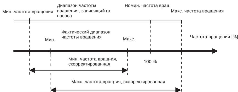
Рис. 120 Установка минимальных и максимальных кривых характеристик в процентах от максимальной производительности.
