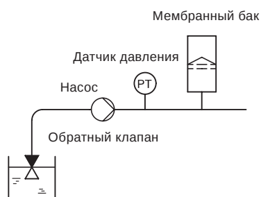
Рис. 86 Расположение обратного клапана и датчика давления в системе, предусматривающей всасывание или работу с отрицательным давлением на входе
